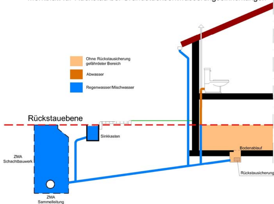
Merkblatt für Rückstau bei Grundstücksentwässerungseinrichtungen
